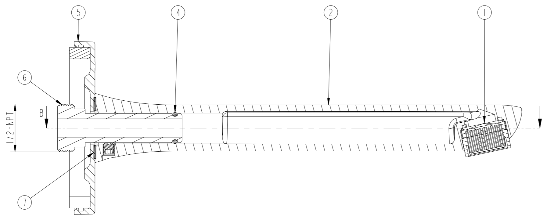
SECTION A-A
