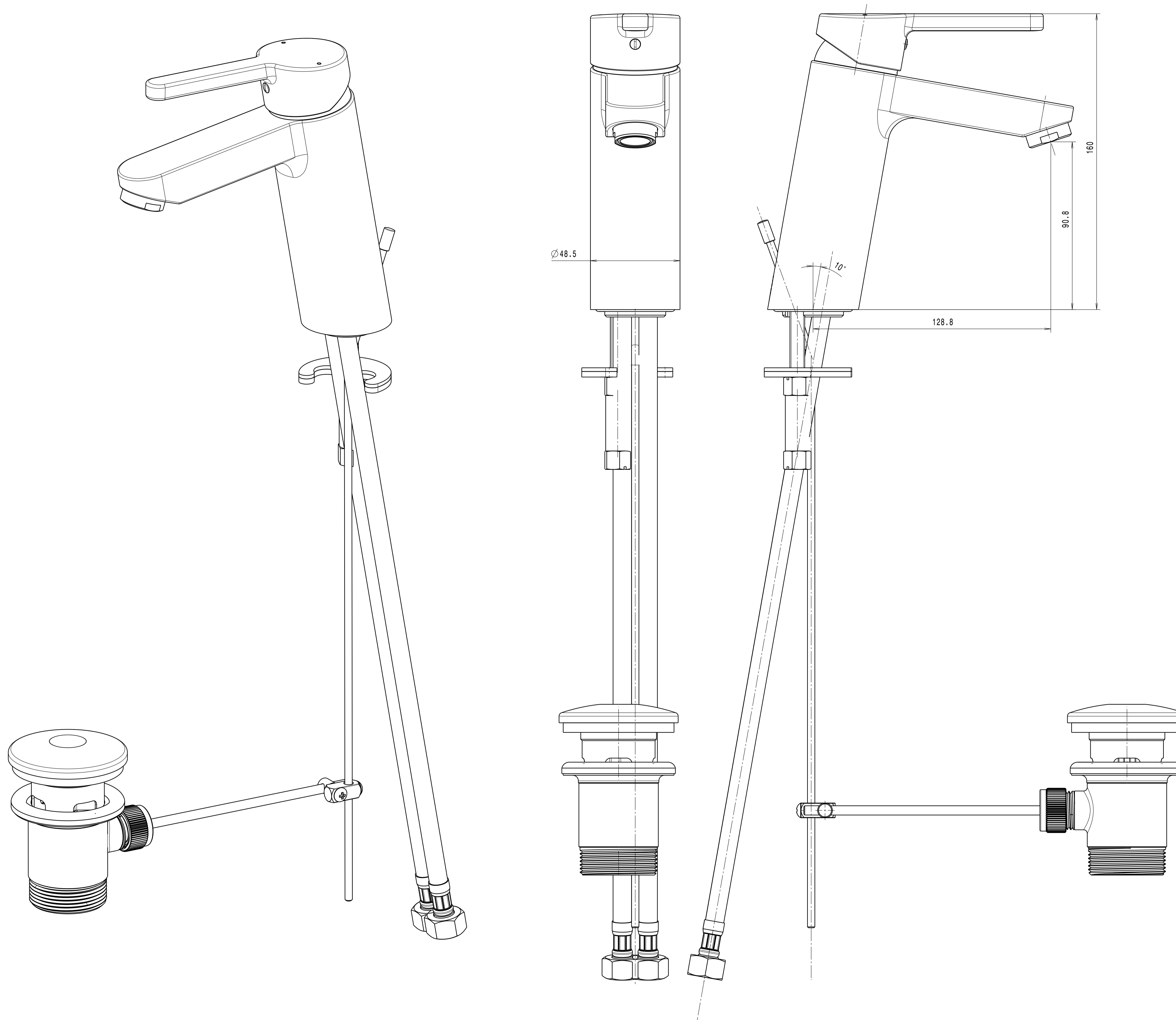
MIRA Einhebelwaschtischarmatur 3.5 MIRA one-hole 3.5 single-lever mixer
