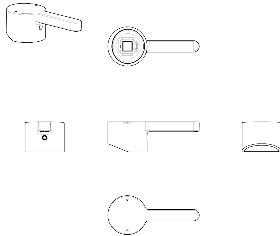
SCALE 1:2
